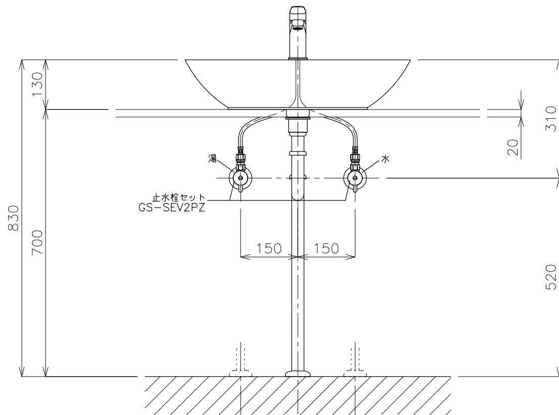
立面図
