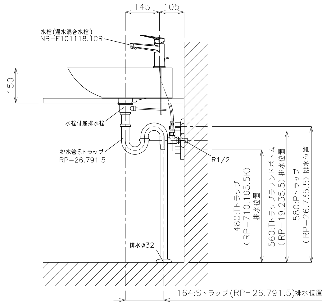
側面図
